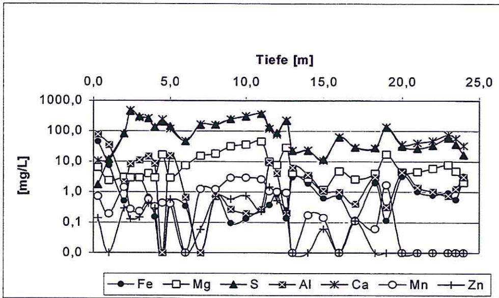
Abb. 7: Analytkonzentrationen [ \text{mg l}^{-1} ] in wäßrigen Eluaten (Einmalelution; DIN 38414)
