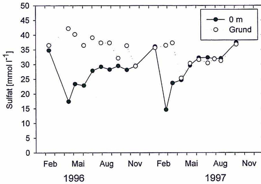
Abb. 2: Jahrgang der Sulfatkonzentration in RS 107 an der Oberfläche und über Grund.
