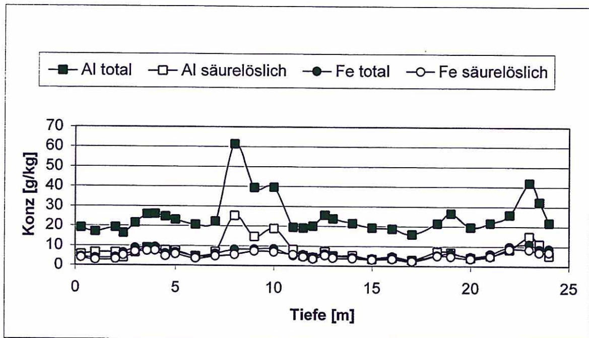
Abb. 4: Teufenabhängigkeit der Konzentrationen für Al und Fe; Vergleich: Totalgehalt (RFA – Daten) und maximal säurelöslicher Anteil
