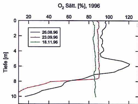
Abb. 13: Ausgewählte Profile der Fluoreszenz und der Sauerstoffsättigung, RL B, 1996
