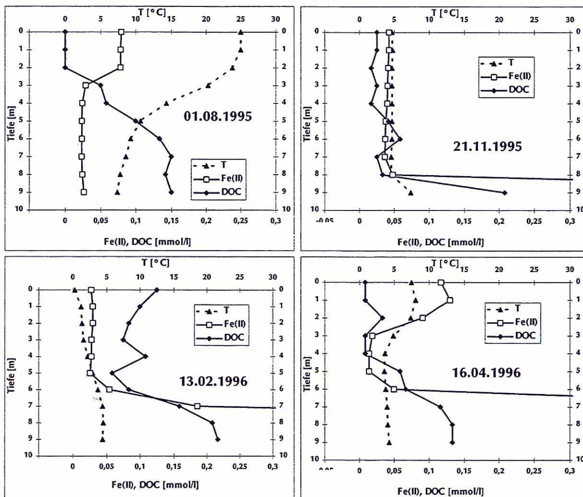
Abb. 4: Temperaturverteilung, Eisen(II)- und DOC-Konzentration in RL 111 zu vier verschiedenen Jahreszeiten
