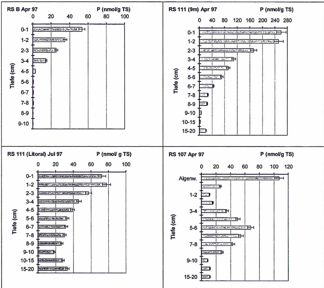
Abb. 2: Mikrobielle Biomasse (als Lipid-Phosphat) in Restseesedimenten. Dargestellt sind die Mittelwerte aus zwei Bestimmungen. Die Fehlerbalken zeigen den prozentualen Variationskoeffizient, bestimmt aus 12 Parallelproben einer Sedimentprobe. Algenw.= Algenwatte
