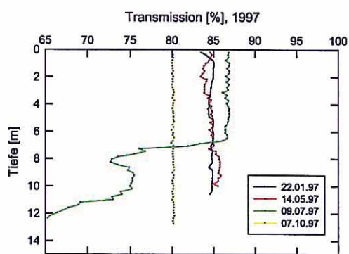
Abb. 14: Ausgewählte Profile der Transmission, RL 117
