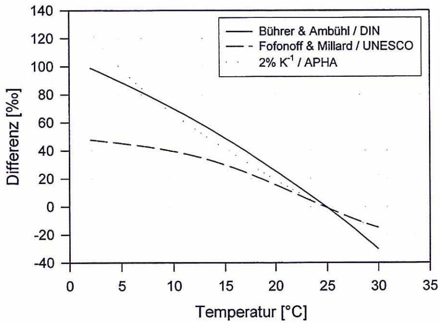
Abb. 20: Relative Differenzen der Temperaturkorrekturfaktoren der elektrischen Leitfähigkeit bezogen auf 25°C für RL107
