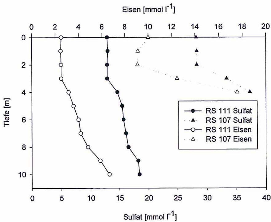
Abb. 3: Vertikale Verteilung der Konzentrationen von Sulfat und Eisen in RS 111 und RS 107 im Sommer 1996.
