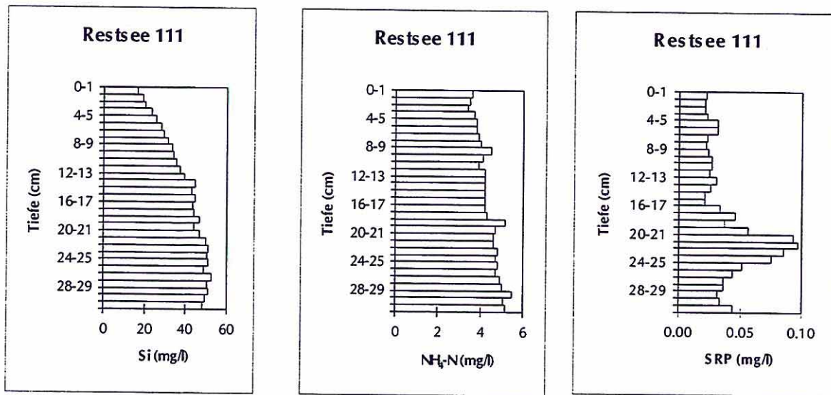
Abb. 6: Tiefenprofile der Nährstoffe Si, NH 4 -N und SRP im Porenwasser von RS-111.
