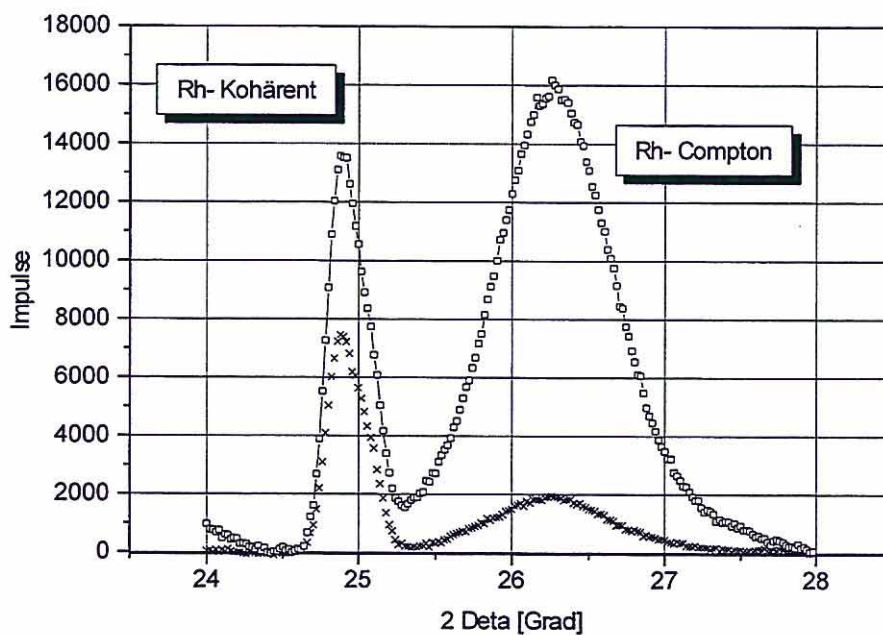
Abb.1: Rh K_{\alpha} Kohärent- und Compton gestreute Strahlung an einem SiO 2 - (□□□) bzw. Fe 2 O 3 - (xxx) Target
