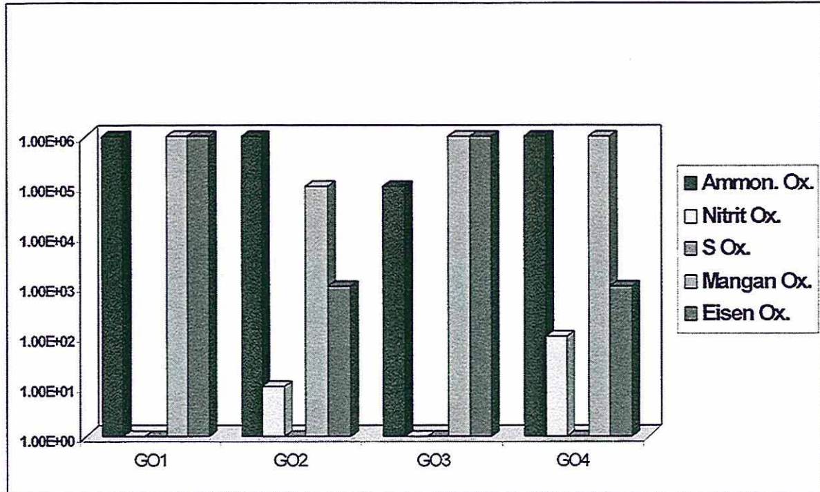
Abb. 1: Verteilung der oxidierenden Bakteriengruppen in den Proben GO1 bis GO4.
