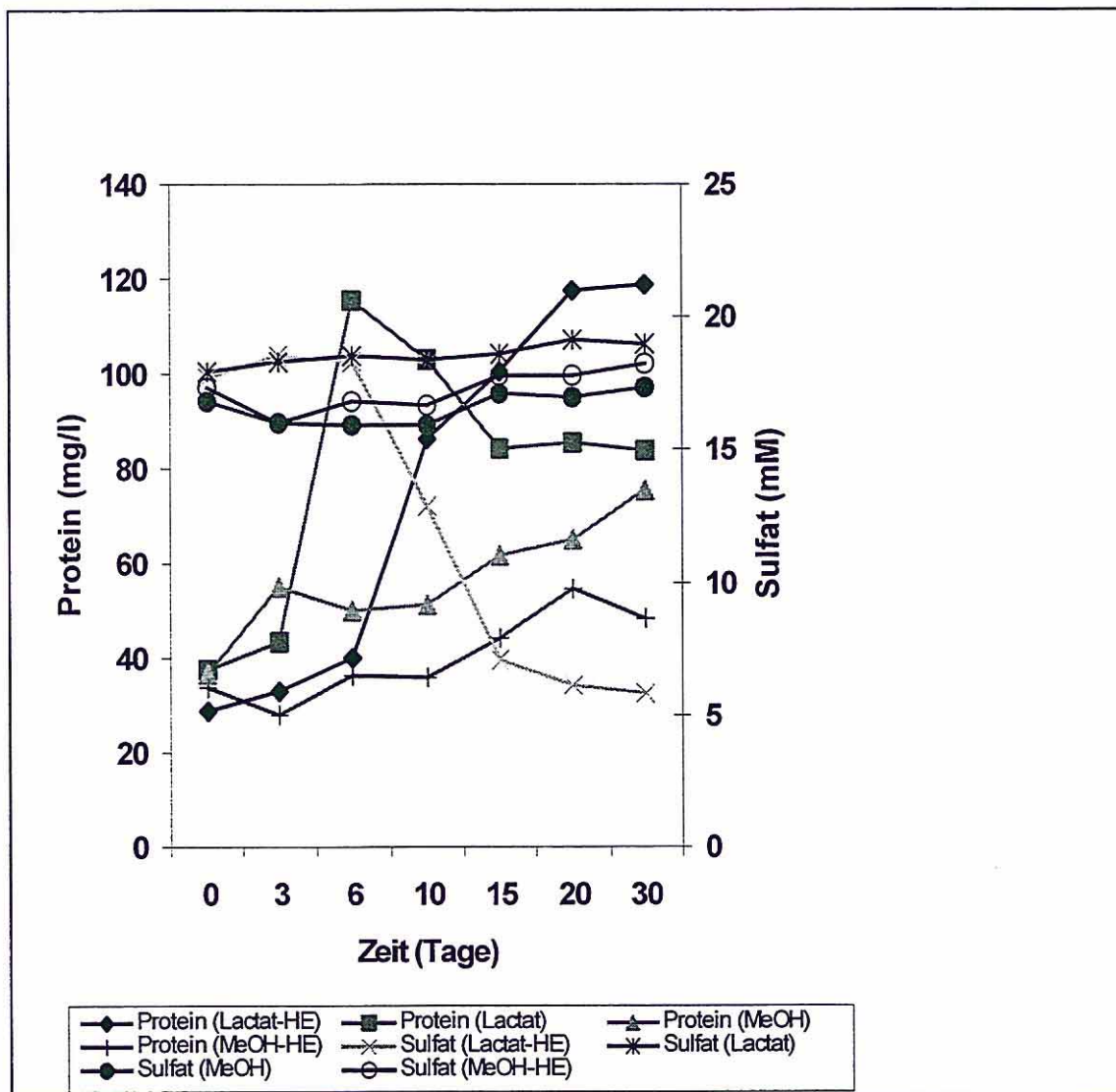
Abb. 3c. Wachstum und Sulfatreduktion der Anreicherungskultur GO3.
