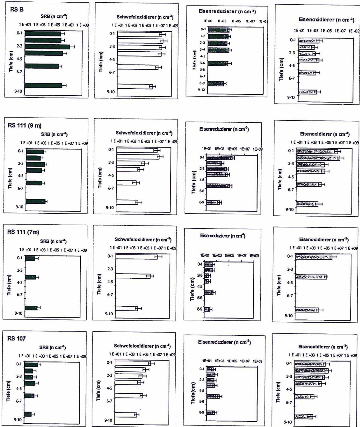
Abb. 6: MPN der sulfatreduzierenden, schwefeloxidierenden und eisenreduzierenden und -oxidierenden Bakterien in den Sedimenten von RS B, RS 111 und RS 107 (April 1997). Fehlerbalken: 95 %-Konfidenzintervall.
