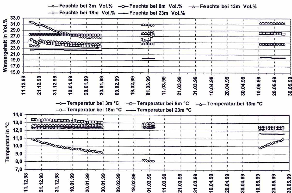
Sickerwasser Grundwasser Meßeinrichtung (SGM) - Sickerwassermeßstelle Goitsche Entwicklung von Substratfeuchte und Temperatur in 5 Meßtiefen (Ungesättigte Zone)
