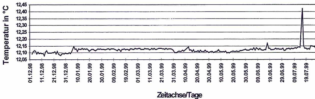
Wasserstand in cm über dem Meßfühler (Meßfühler 27,1m unter GO) Temperatur des Grundwassers in dieser Tiefe Grundwassermeßstelle Goitsche des SGM Meßergebnisse des Multisensormeßsystems (MSN)
