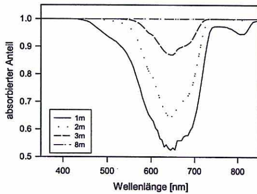
Abb 17: Unterwasserlichtspektren in versch. Tiefen in RS 111 am 20.8.97
