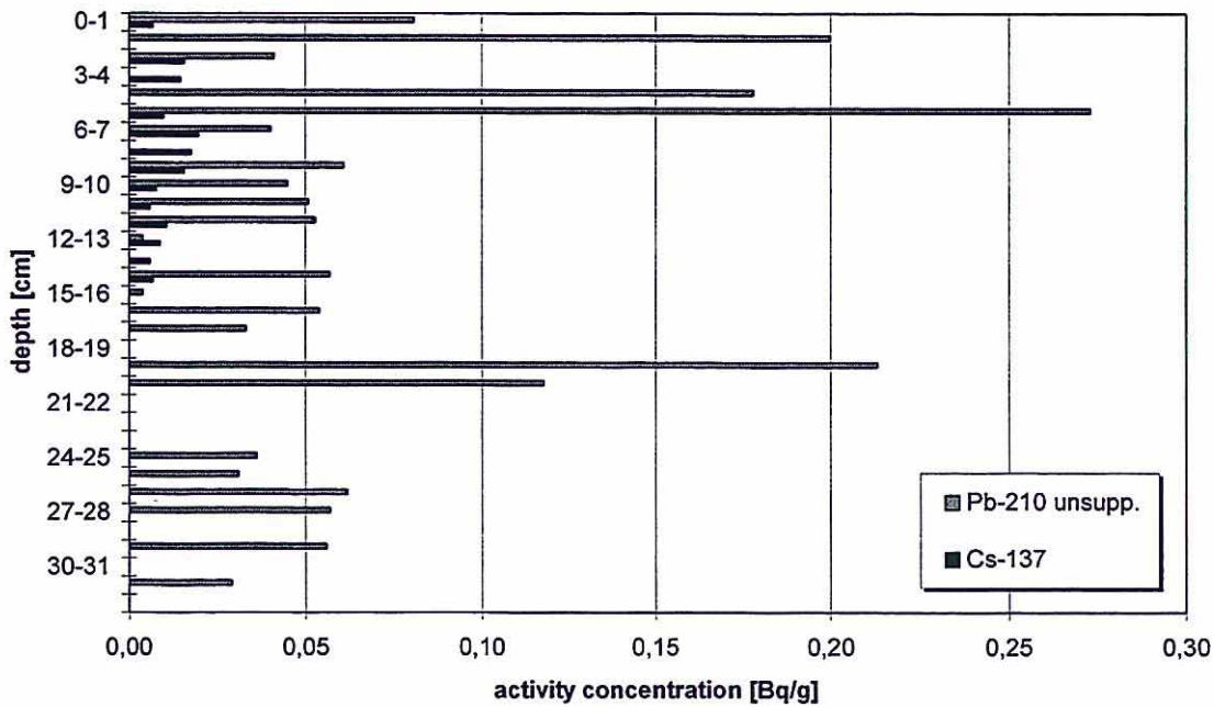
Abb. 4: Tiefenverteilung von 137 Cs und 210 Pb im Sedimentkern Nr. 18, RL 107
