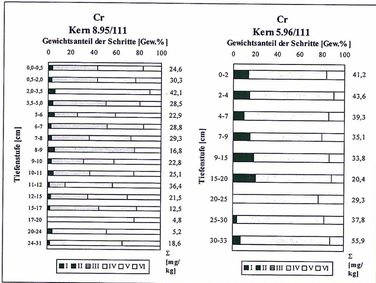
Abb. 3: Bindungsforminventar von Cr in Kern 8.95/111 und Kern 5.96/111 I: adsorptiv, II: karbonatisch, III: leicht reduzierbar, IV: weniger leicht reduzierbar, V: sulfidisch/organisch, VI: residual
