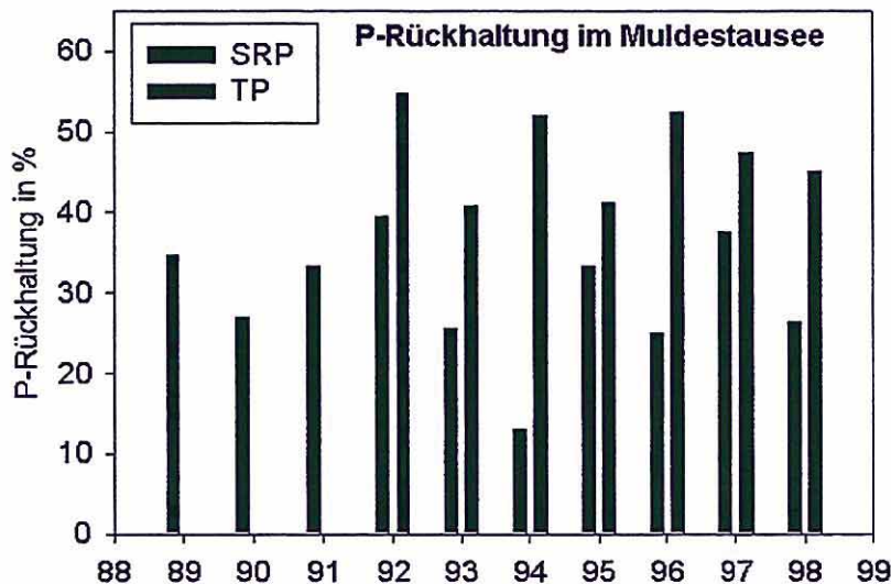
Abb. 2: Phosphorrückhaltung im Muldestausee in den Jahren 1989-98 (Vergleich der Mittelwerte der Phosphorkonzentrationen am Zu- und Ablauf; SRP-gelöster, molybdatreaktiver Phosphor, TP-Gesamtposphor). Für die einzelnen Jahre standen je 16-26 Werte zur Verfügung (Datenquelle: Gewässergüteberichte des Landesamtes für Umweltschutz Sachsen-Anhalt).
