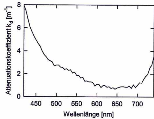
Abb. 18: Wellenlängenabhängigkeit von k_d aus dem Lichtspektrum in 1 m Tiefe im RS 111
