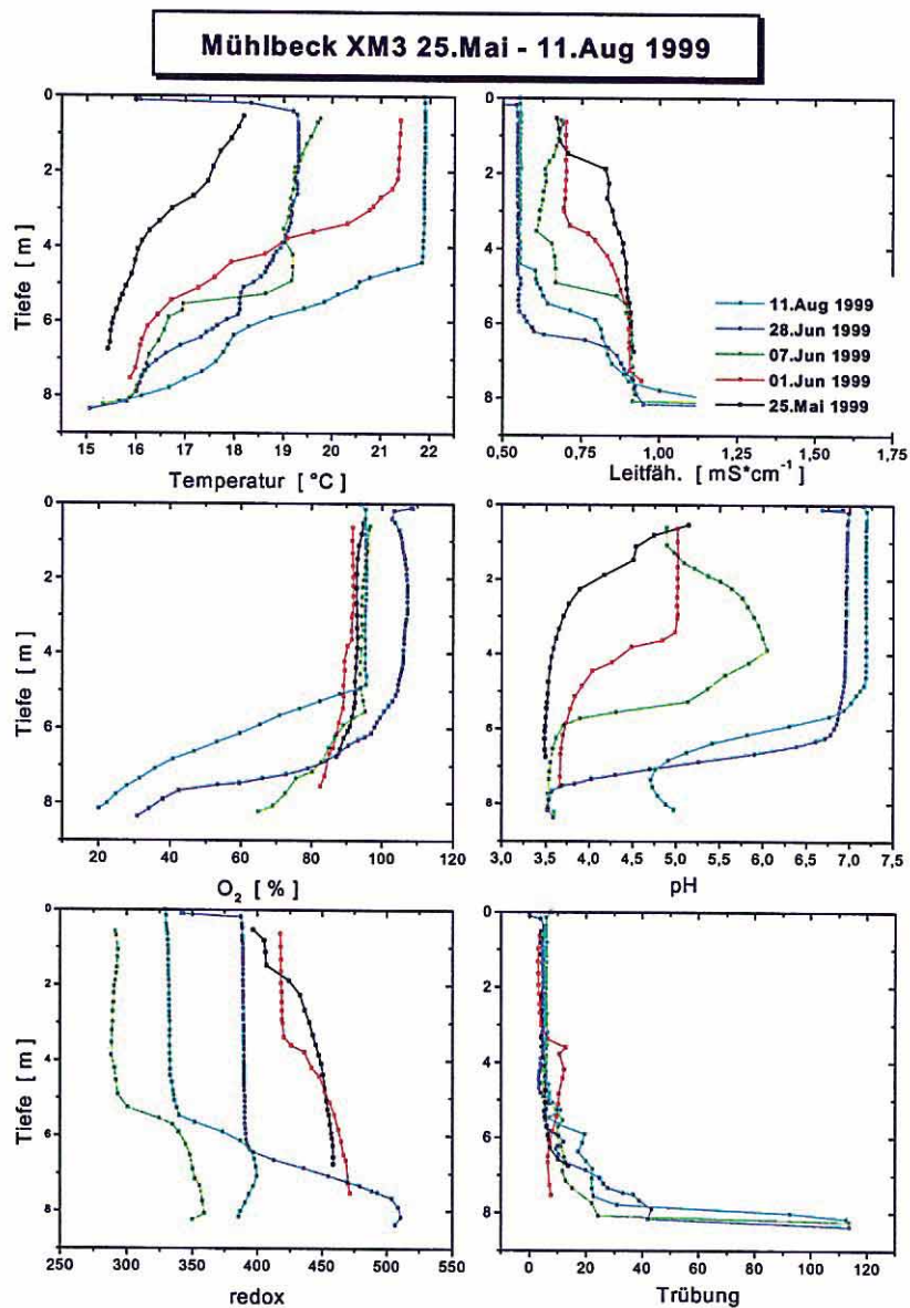
Abbildung 3: Profilmessungen in Restsee Mühlbeck an der Probenahmestelle XM3 für physikalische und physikalisch-chemische Messgrößen über die thermische Schichtungsphase in der Zeit vom 25.Mai 1999 bis zum 11.Aug 1999
