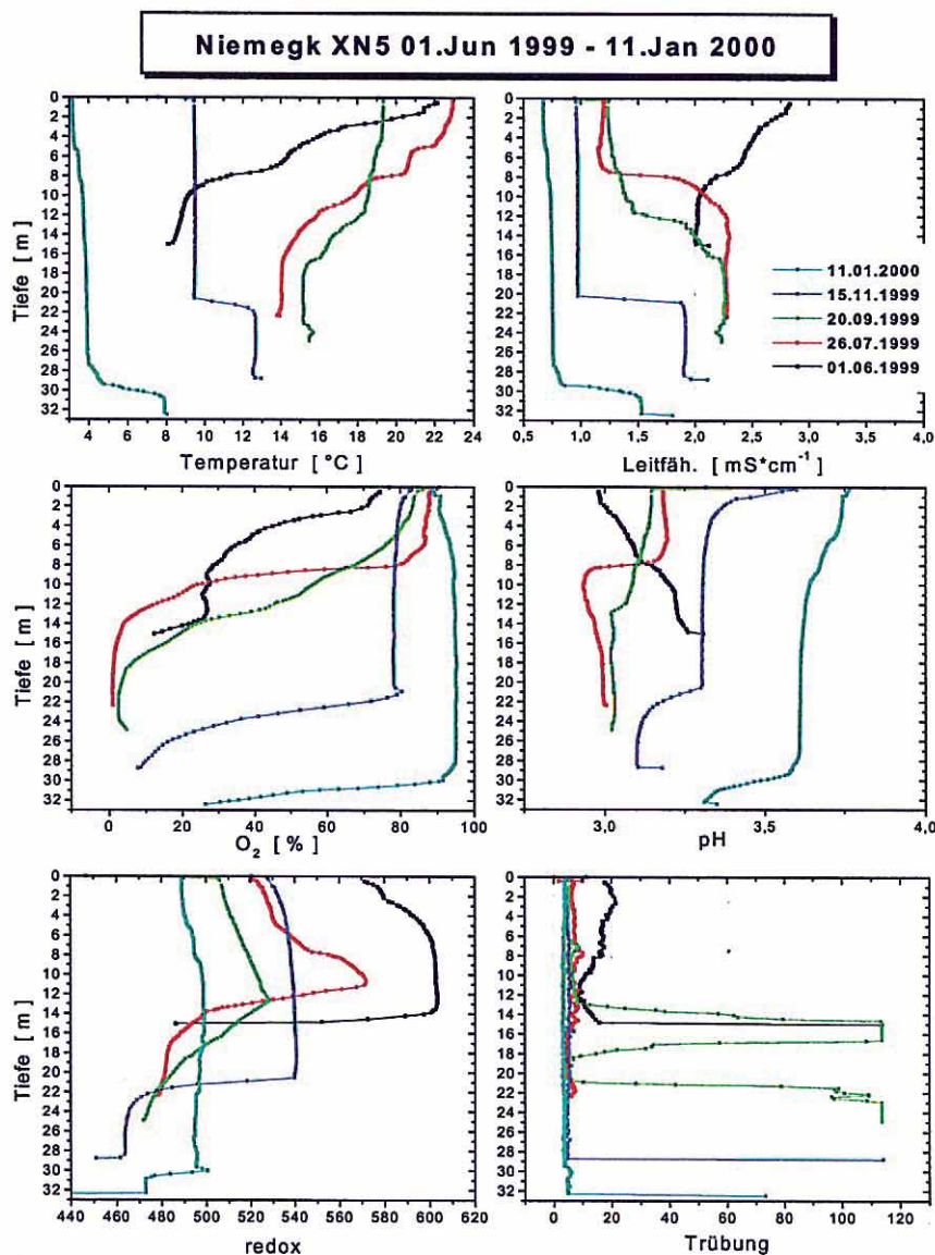
Abbildung 5: Profilmessungen im Restsee Niemegk an der Probenahmestelle XN5 für physikalische und physikalisch-chemische Messgrößen in der Zeit vom Einsetzen des Überlaufs von Mühlbeck nach Niemegk bis zum Einsetzen des Überlaufs von Niemegk nach Bärenhof
