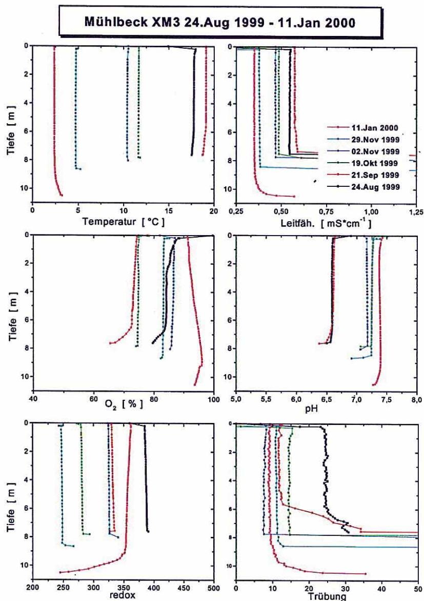
Abbildung 4: Profilmessungen in Restsee Mühlbeck an der Probenahmestelle XM3 für physikalische und physikalisch-chemische Messgrößen nach der thermischen Schichtungsphase in der Zeit vom 24.Aug 1999 bis 11.Jan 2000
