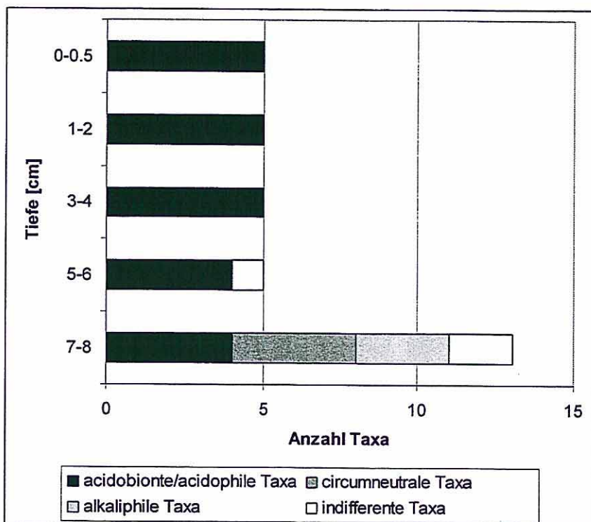
Abb. 2: Anzahl der acidobionten/acidophilen, circumneutralen, alkaliphilen und indifferenten Diatomeen-Taxa in einem Bohrkern aus dem Restsee 117, Lausitz.
