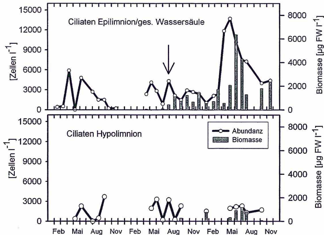
Abbildung 3: Zellichten und Biomassen der Planktonciliaten im Restsee B von 1995-1997. Der Pfeil markiert das erste Auftreten von Stentor amethystinus .
