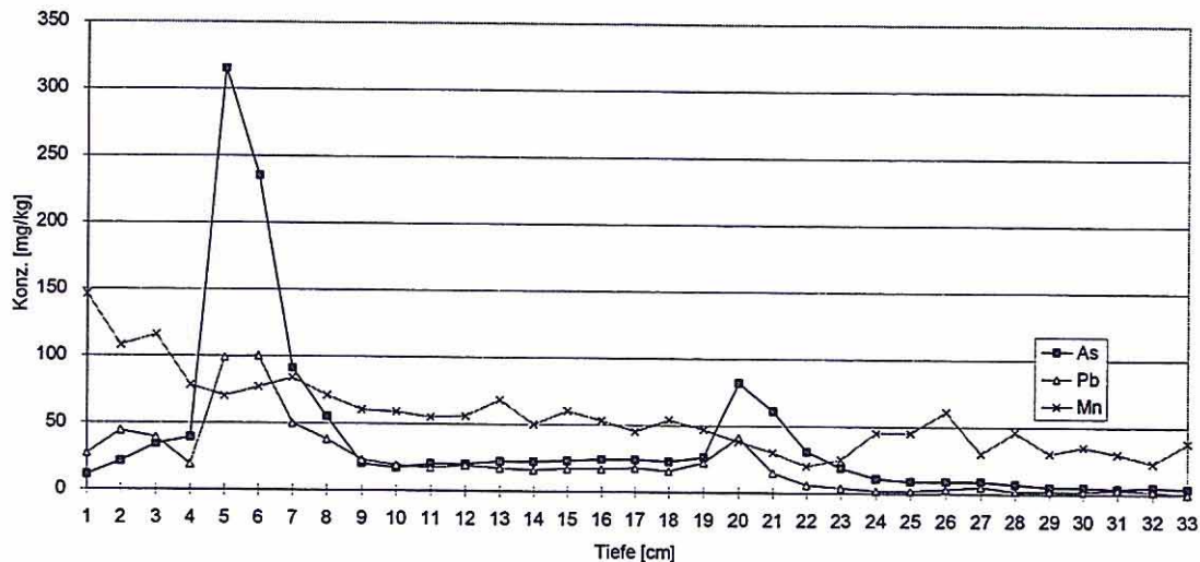
Abb. 6: Tiefenverteilung der Spurenelemente Mn, As und Pb am Beispiel des Sedimentkernes K18 von ML 107.
