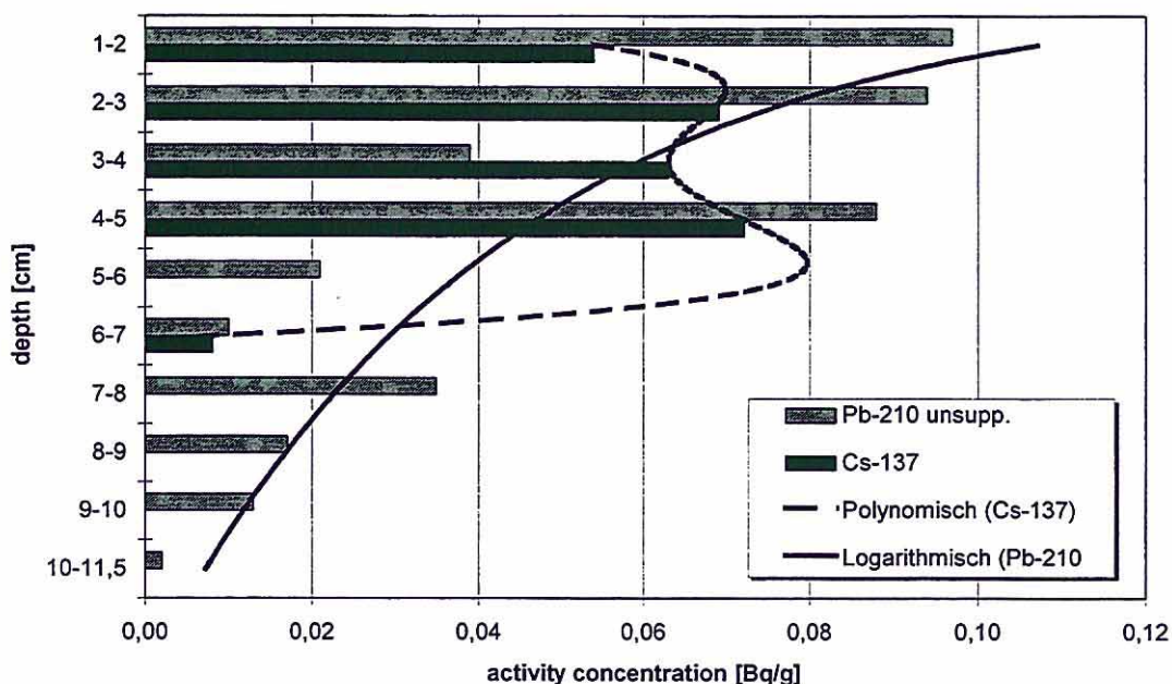
Abb. 2: Tiefenverteilung von ^{137}\text{Cs} und ^{210}\text{Pb} im Sedimentkern Nr. 5, RL B
