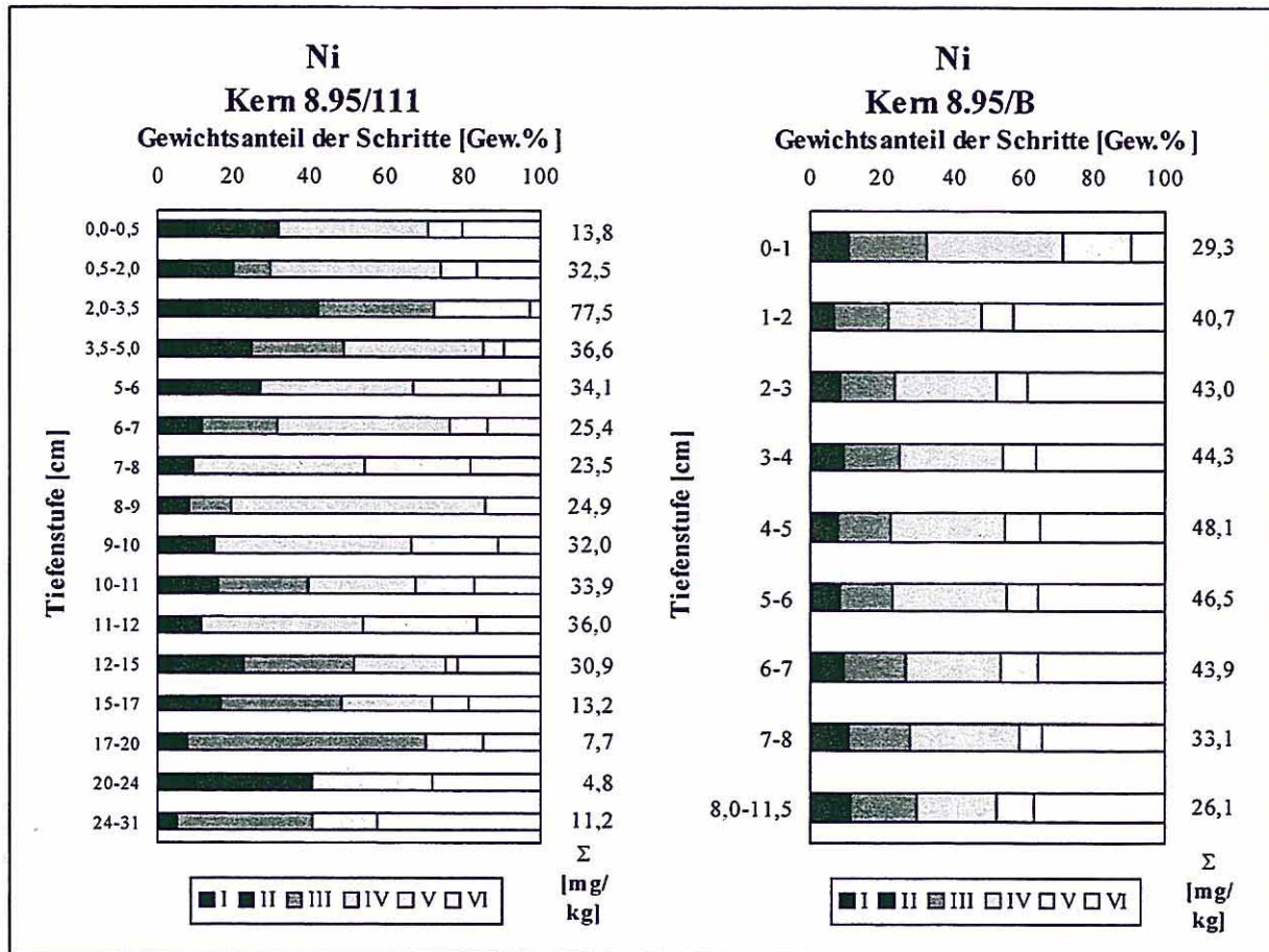
Abb. 2: Bindungsforminventar von Ni in Kern 8.95/111 und Kern 8.95/B I: ádsorptiv, II: karbonatisch, III: leicht reduzierbar, IV: weniger leicht reduzierbar, V: sulfidisch/organisch, VI: residual
