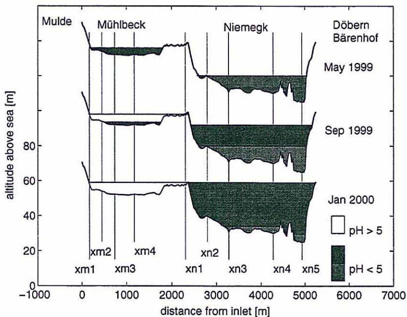
Abbildung 7: Skizzierte Schichtung in den Seen Mühlbeck und Niemegek. Auftragung der geographischen Höhe gegen Distanz vom Flutungszulauf entlang des Talwegs in Abbildung 1. Zwei verschieden schattierte Wasserkörper in einem Seebecken sind durch eine andauernde Schichtung voneinander getrennt und erfahren nur einen geringen Austausch untereinander. Die beiden oberen Graphiken sind gegen die mNN-Skala um 40m bzw. 80m verschoben.
