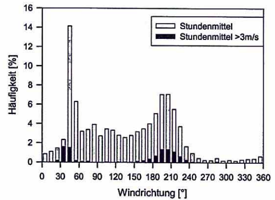
Abb. 19: Häufigkeitsverteilung der Stundenmittel der Windrichtung auf RS 111
