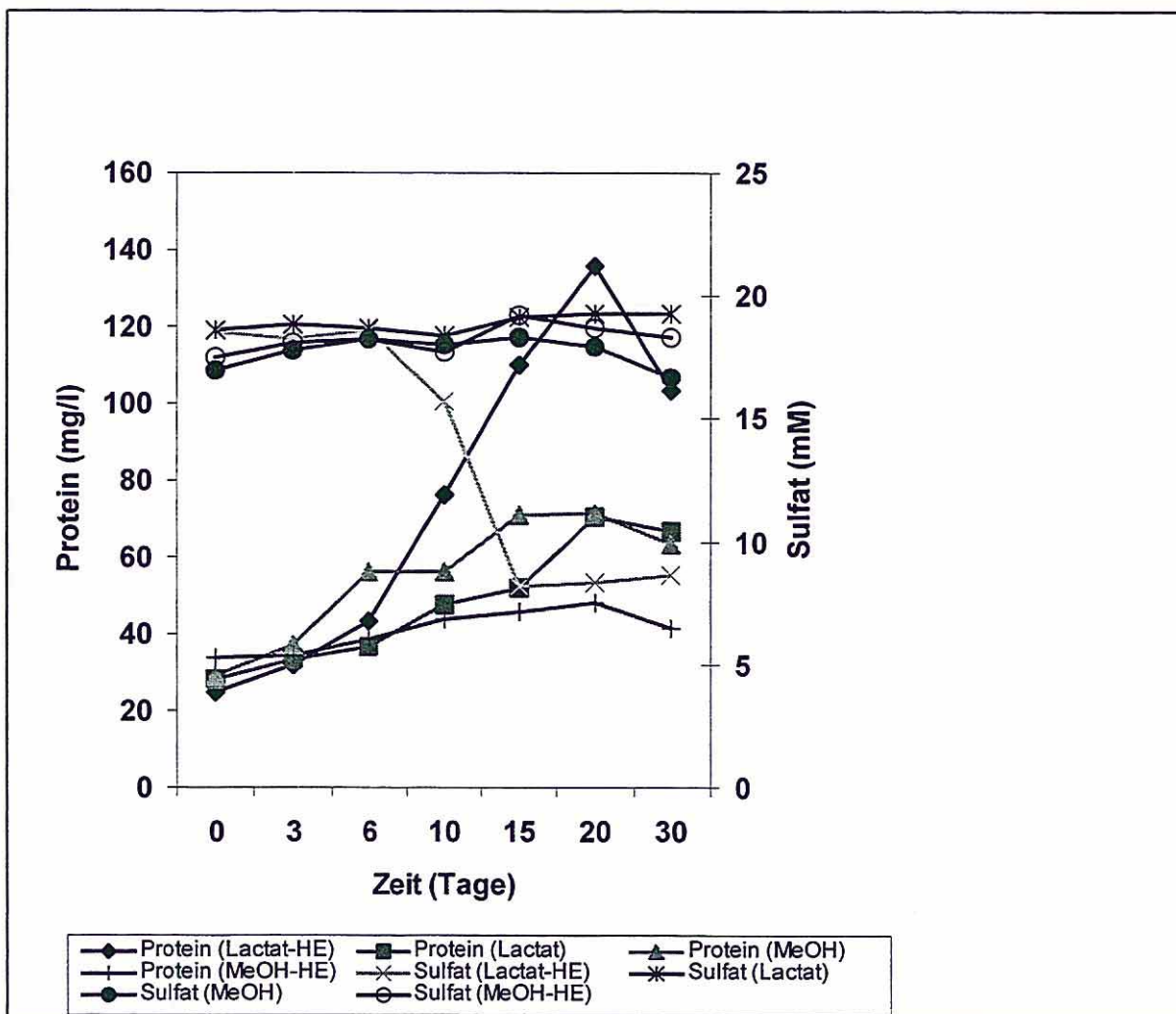
Abb. 3a. Wachstum und Sulfatreduktion der Anreicherungskultur GO1.
