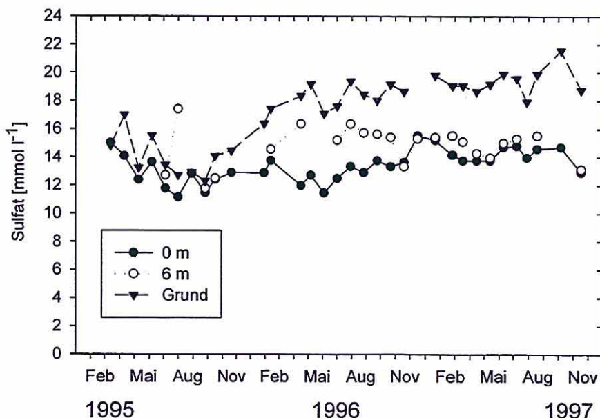
Abb. 1: Jahresgang der Sulfatkonzentration in RS 111 an der Oberfläche, in 6 m Tiefe und über Grund.
