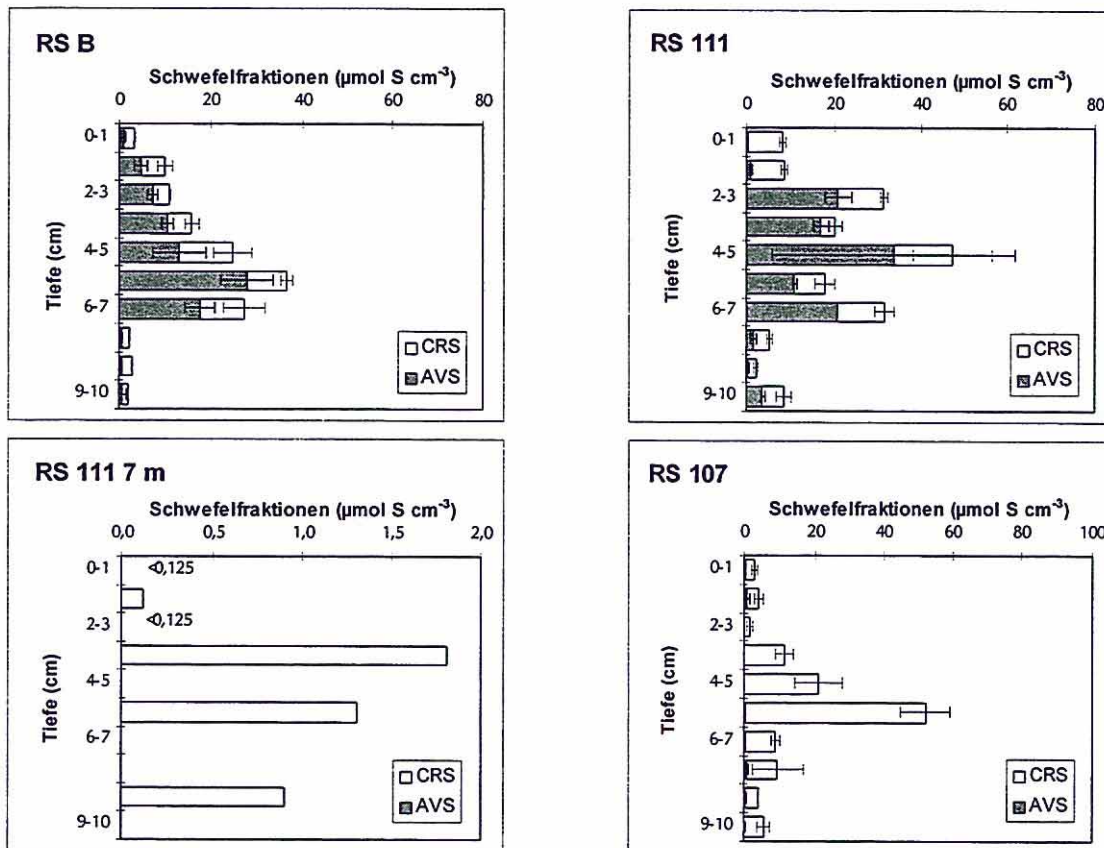
Abb. 3: Verteilung der Schwefelverbindungen (AVS: säureflüchtige und CRS: chromreduzierbare Anteile) in den Sedimenten (April 1997). Mittelwerte von zwei Parallelen, RS 111 (7m) Einfachbestimmung
