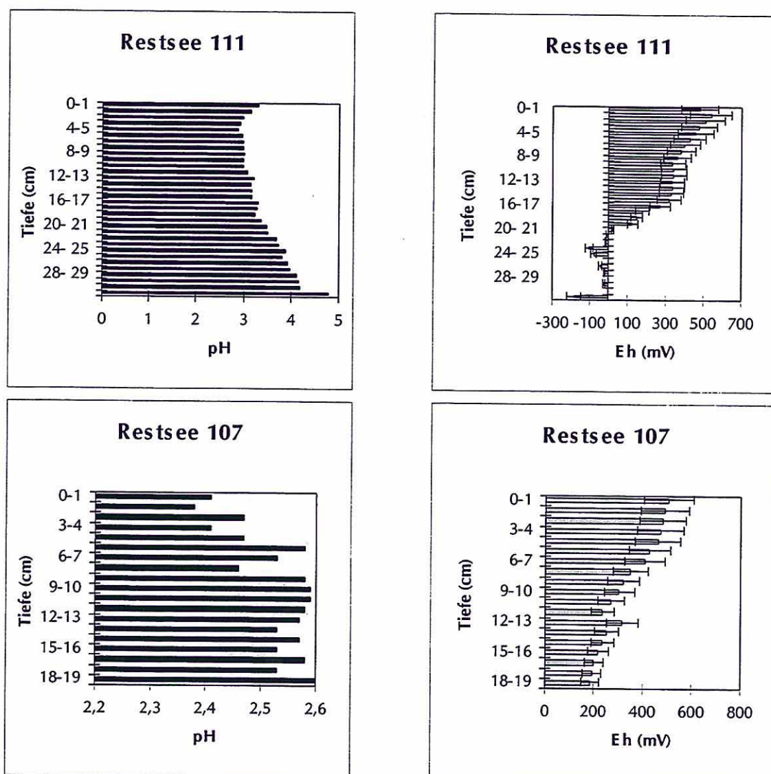
Abb. 1: pH- und Eh-Tiefenprofile in Sedimenten von RS-B, RS-111 und RS-107.
