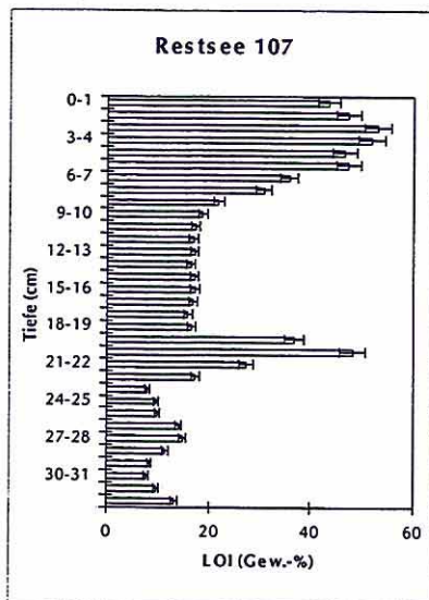
Abb. 4ff: Sediment-Tiefenprofile von Haupt-, Neben- und Spurenelementen sowie Glühverlust (LOI) in RS-107.
