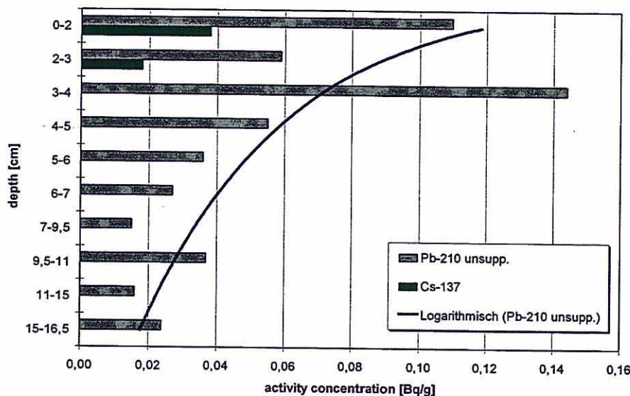
Abb. 1: Tiefenverteilung von ^{137}\text{Cs} und ^{210}\text{Pb} im Sedimentkern 4, RL B
