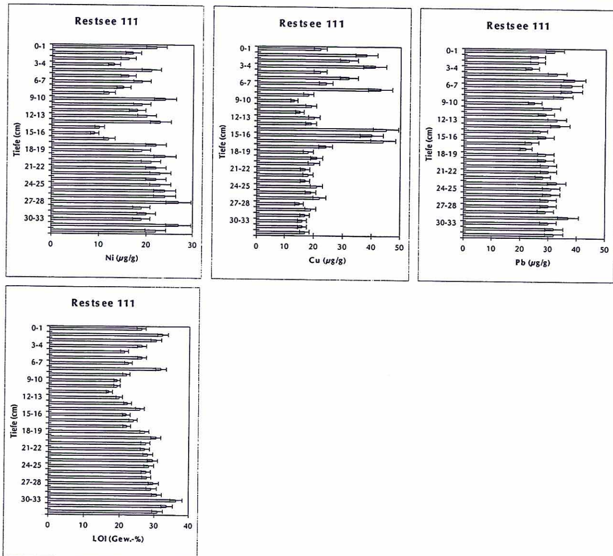
Abb. 3ff: Sediment-Tiefenprofile von Haupt-, Neben- und Spurenelementen sowie Glühverlust (LOI) in RS-111
