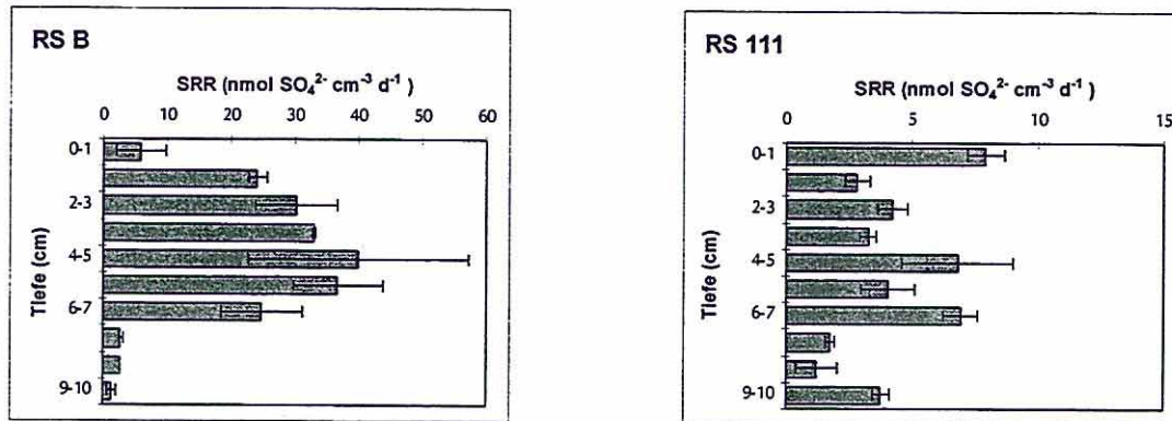
Abb. 3.3.2: Sulfatreduktionsraten in den Sedimenten von RS B und RS 111 (April 1997). Mittelwert aus zwei Parallelen
