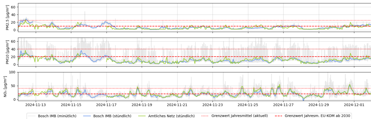
Abbildung 3: PM 2.5 , PM 10 und NO 2 [µg/m 3 ] Messungen verschiedener Sensoren an der amtlichen Luftgütemessstation in Leipzig Mitte vom 12.11.24 – 02.12.24. Im Vergleich sind die Zeitreihen der Bosch Sensorik (IMB) und der amtlichen Station gegenübergestellt.
