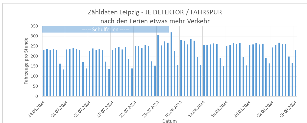
Abbildung 6: Durchschnittliche Tageszählwerte je Detektor und Fahrspur über alle verfügbaren Zählwerte.
