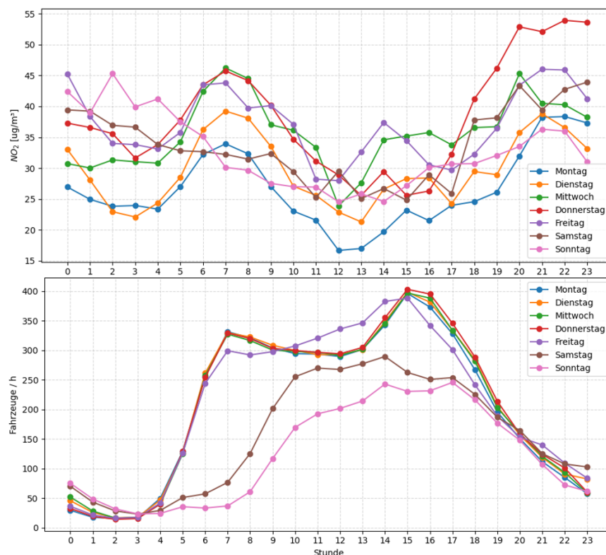
Abbildung 8: Typischer Wochenverlauf (gemittelt) der Luftqualität ( \text{NO}_2 , oben) und der Fahrzeuge pro Stunde (unten). Die gemittelten Werte beziehen sich auf einen Zeitraum vom 10. Juni bis 5. August 2024.
