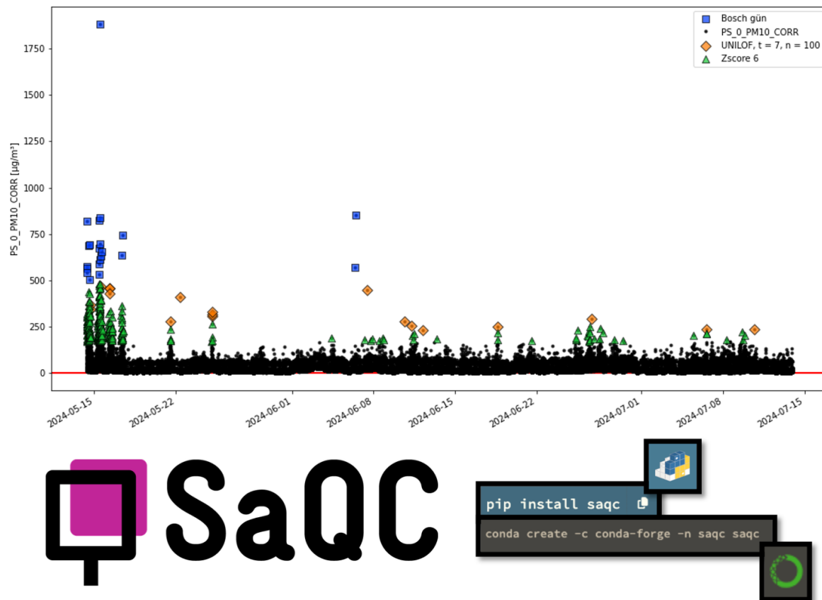
Abbildung 4: Automatisierte Qualitätskontrolle von Zeitreihendaten mit Hilfe von SaQC am Beispiel einer PM_{10} - Messreihe im Sommer 2024. Beispielhaft wurden Ausreißer mit Hilfe verschiedener parametrisierter statistischer Tests markiert. Die statistischen Tests sind in der Software SaQC umgesetzt und können durch den Anwender auf den jeweiligen Datensatz zugeschnitten werden. Im operationellen Betrieb der UFZ Infrastruktur geschieht die QC anschließend voll automatisch und kontinuierlich.
