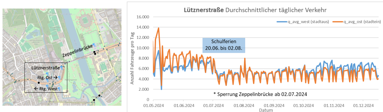
Abbildung 7: links: Kartenausschnitt Quarterback Arena, Zeppelinbrücke, Lütznerstraße., rechts: Entwicklung der Tageszählwerte in der Lütznerstraße je Fahrtrichtung im Verlauf der Monate.
