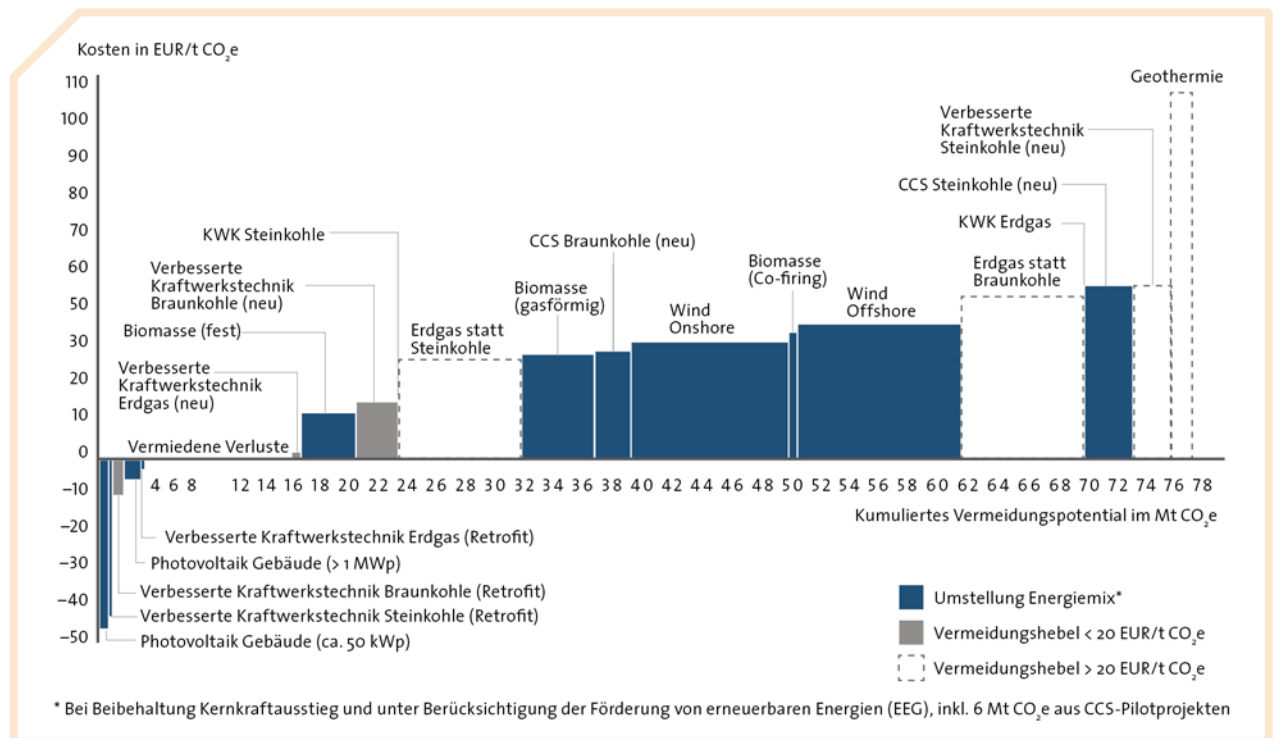
ABBILDUNG 2.9 ▶ Vermeidungskostenkurve im Energiesektor für Deutschland 2020.
