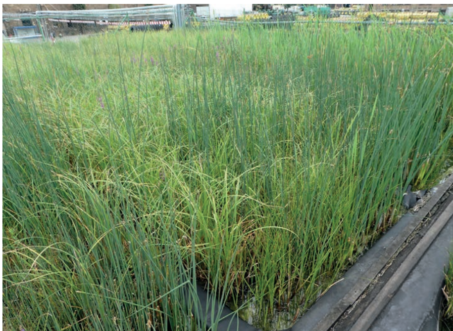
Abb. 2: Sumpfpflanzendach zur Prozesswasserbehand- lung der Firma John Deere in Mannheim 2018 (Foto: A. Zehnsdorf).
