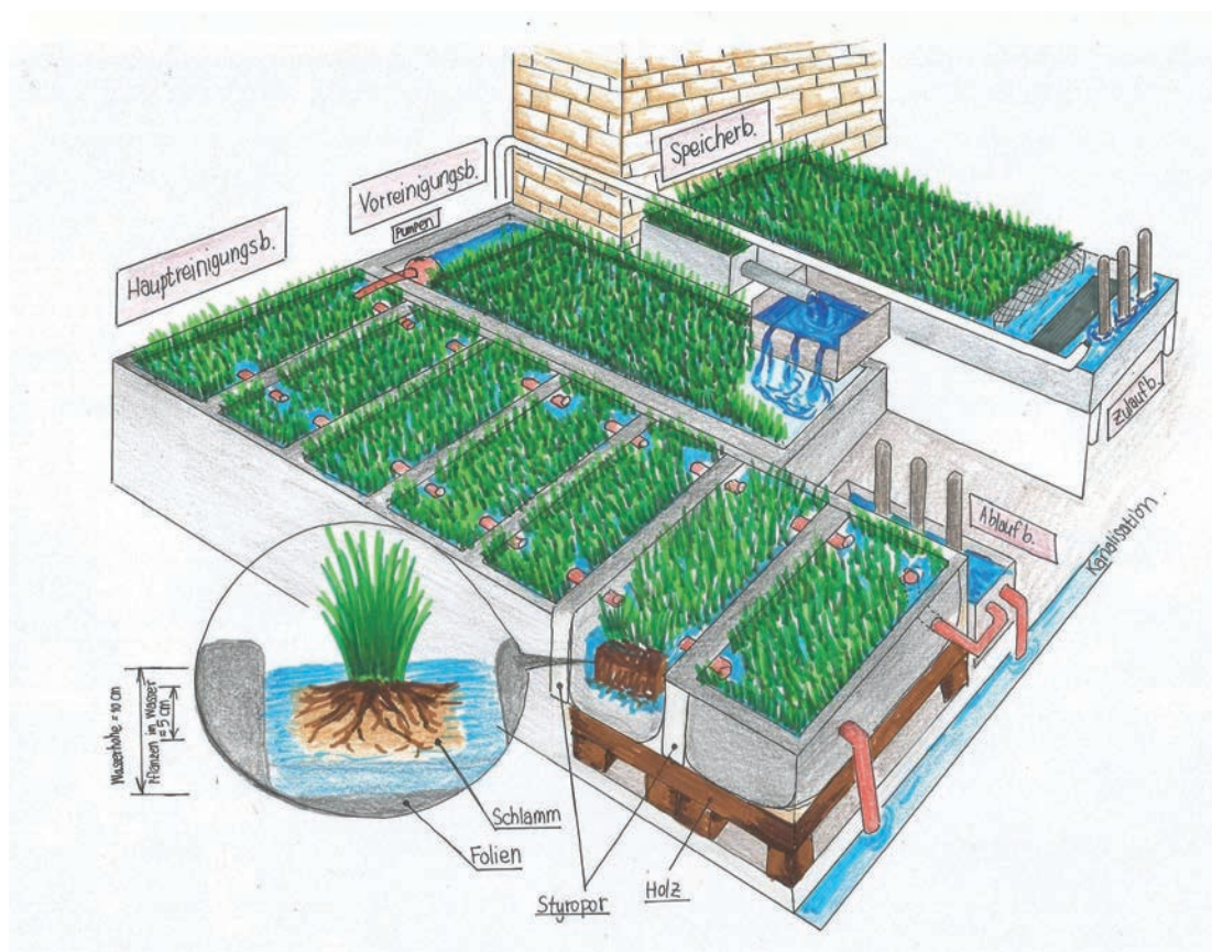
Abb. 2: Schnittzeichnung der Anlage (Quelle: John Deere).
