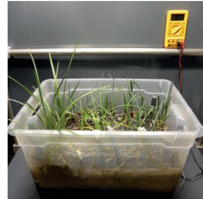
Abb. 2: Versuchsaufbau mit der Sumpfschilf ( Carex acutiformis ) als bepflanzte mikrobielle Brennstoffzelle (Grafik und Foto: A. Zehndorf).
