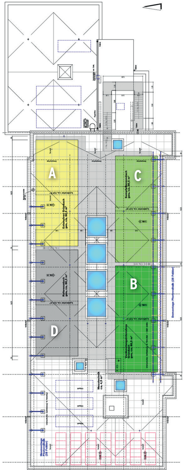
Abb. 7: Detailzeichnung Dachdraufsicht Pilotanlage Forschungsgründach (Zeichnung: BAUPLAN).
