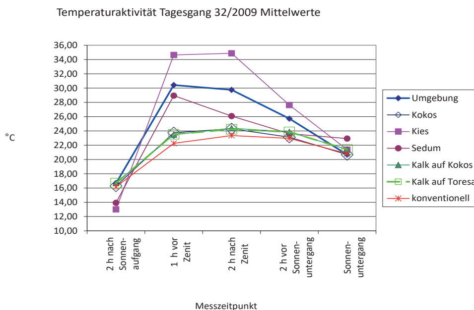
Abb. 23: Mittlerer Tagesgang der Temperatur unter den Filtertablets in Woche 32, 2009
