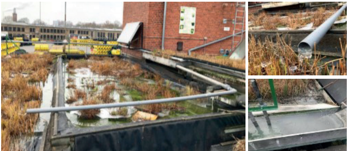
Abb. 5: links: Einstellung des Notfallrohres vom Speicherbecken zum sechsten Becken des Hauptreinigungsbeckens; Fotografiert am 23.01.2019 rechts oben: Das gebildete Eis im Notfallrohr bei Temperatur -1 °C; Fotografiert am 24.01.2019 rechts unten: Das gefrorene Abwasser im Zulaufbecken bei Temperatur unter -1 Grad; Fotografiert am 24.01.2019 (Fotos: John Deere).
