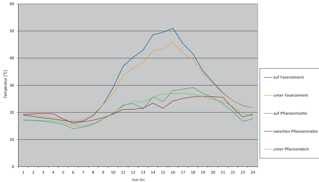
Abb. 7: Tagesgang der Temperaturverläufe auf und unter dem Normaldach sowie zwischen Wurzelschutzfolie und Faserzementdach und unter dem Sumpfpflanzendach, gemessen am 30.7.2006.
