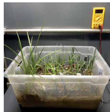
Abb. 2: Versuchsaufbau mit der Sumpfsegge ( Carex acutiformis ) als bepflanzte mikrobielle Brennstoffzelle (Grafik und Foto: A. Zehndorf).
