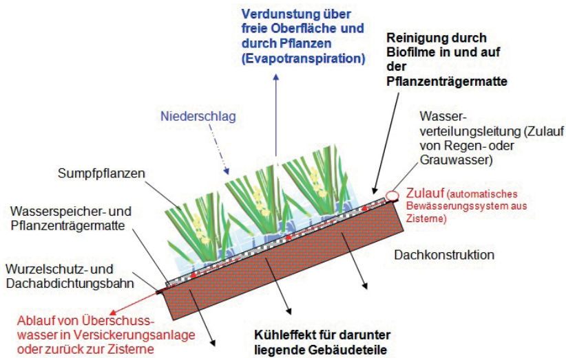
Abb. 3: Aufbau eines Sumpfpflanzendaches (Quelle: M. Blumberg).
