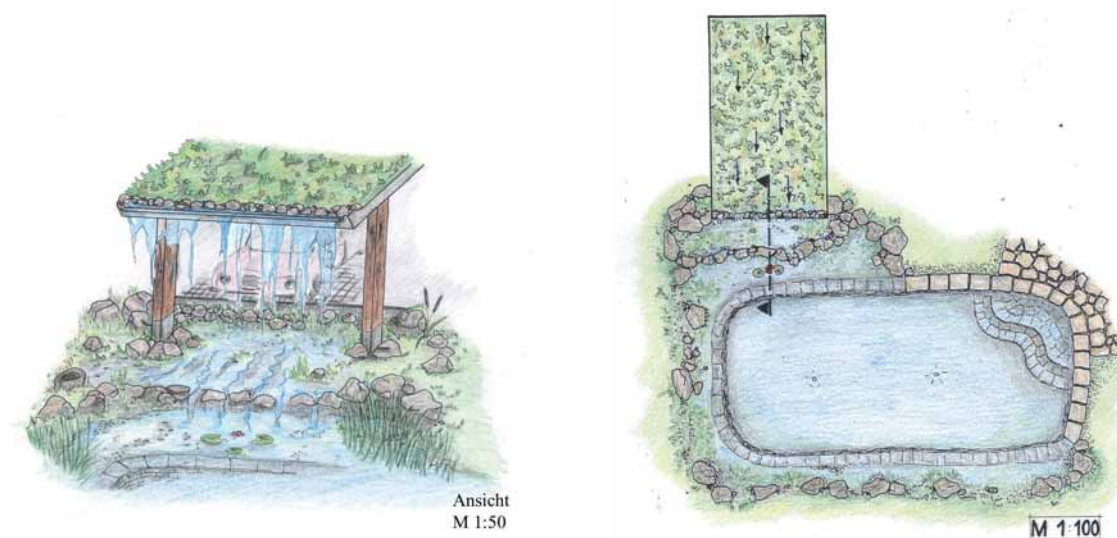
Abb. 1: Carport mit Dachgarten-Filter am Schwimmteich, Ansicht und Draufsicht (Zeichnung: C. Weinreich, HS Anhalt).
