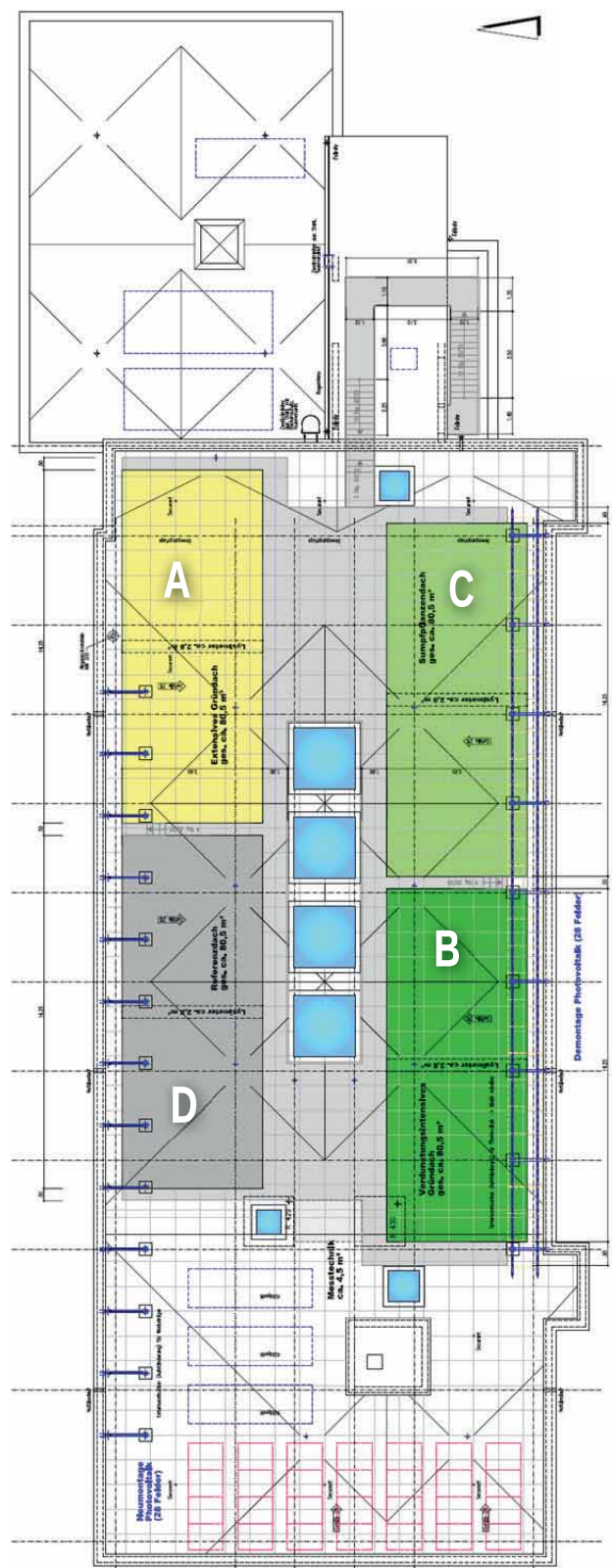
Abb. 7: Detailzeichnung Dachdraufsicht Pilotanlage Forschungsgründach (Zeichnung: BAUPLAN).
