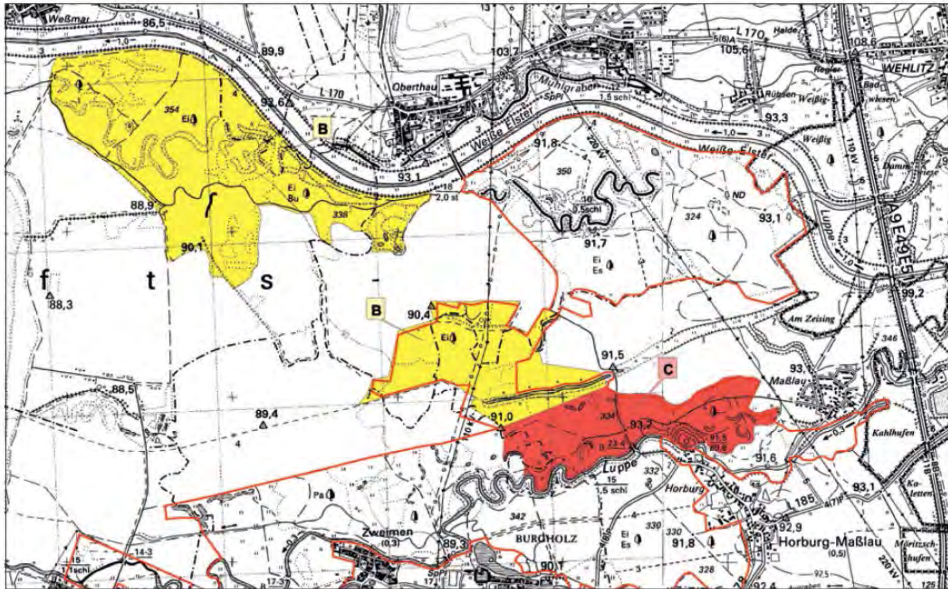
Abb. 4.3-17: Bewertung des Erhaltungszustandes der Teilpopulation von E. matura im FFH-Gebiet 0143.
